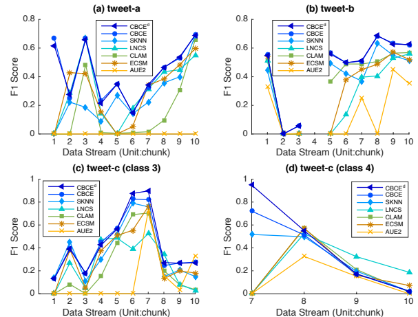
Fig. 9. F1 scores on the tweet streams.
